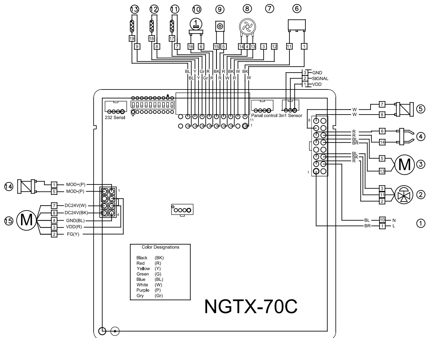
Рисунок 12. Схема электрическая.
